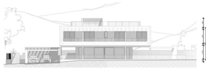
ALZADO SURESTE
