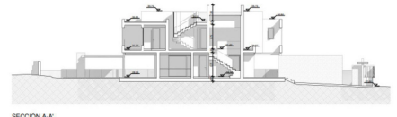
SECCION A-A'
