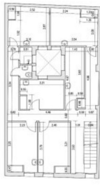
PLANTA PRIMERA
