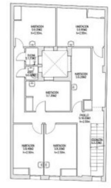
PLANTA PRIMERA SUPERFICIE DEL TOTAL 13.84 M 2 SUPERFICIE CONSTRUIDA 10.36 M 2
