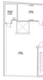
PLANTA CUBIERTA SUPERF. DEL TOTAL 18,40 m 2 SUPERF. CONSTR. 18,73 m 2
