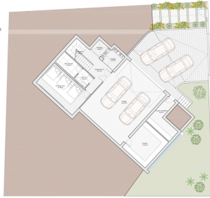
PLANTA SOTANO
