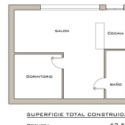
DISTRIBUCION COCHERA Y APARTAMENTO A3 1/125
