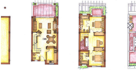
0_ PLANTA BAJA PLANTA PRIMERA PLANTA
