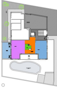
DISTRIBUCIÓN - P0
