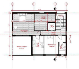
PLANTA PRIMERA
